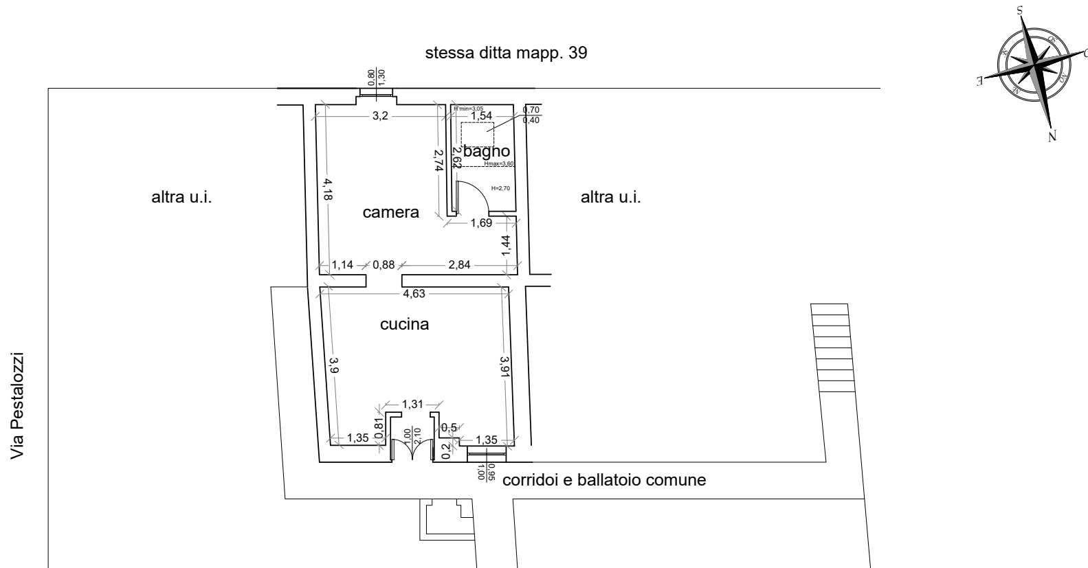
STATO DI PROGETTO PIANO PRIMO H=2,68
